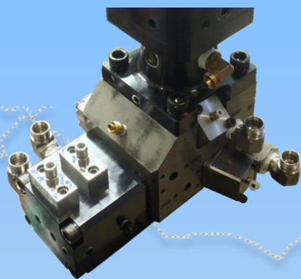
高圧ミキシングヘッド
